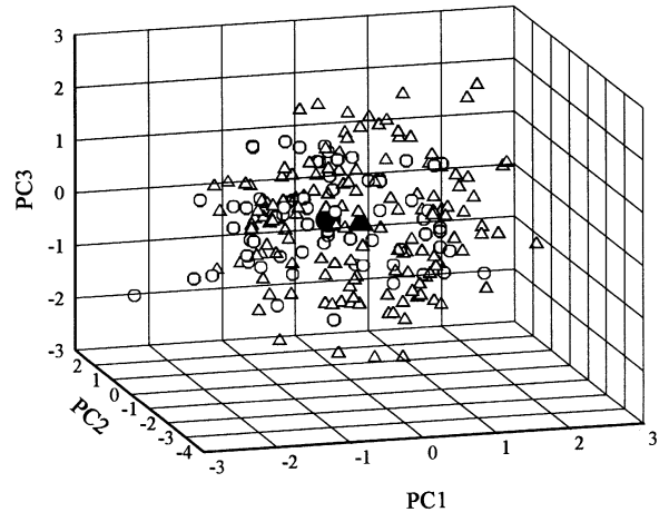
图 2 虎纹蛙两性成体 10 个形态特征的前 3 个主成分荷载因子的分布图
