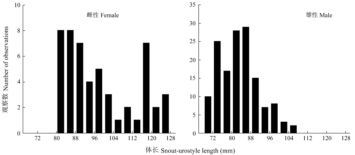
图 1 虎纹蛙成体体长频次分布
